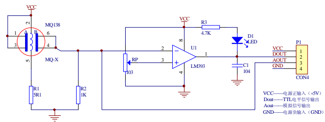
MQ138甲醛气体检测传感器原理图
